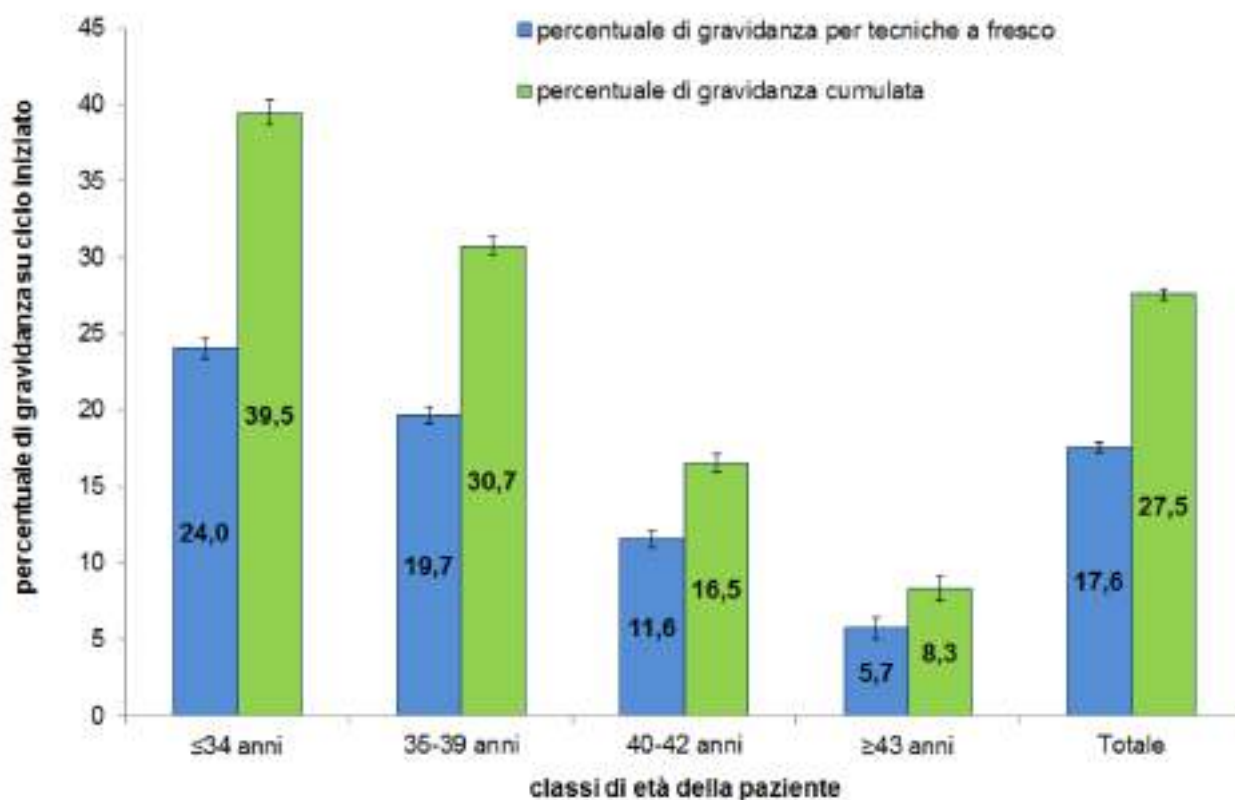
Figura 1: Distribuzione delle probabilità di gravidanza cumulative (e relativi intervalli di confidenza al 95%) per ciclo iniziato con ovociti propri per classe di età (Dati Registro PMA – 2017). Disponibile a:
